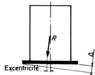
Tassement différent sous le radier, dû au terrain de résistance inégale : déversement du bâtiment et excentricité de la résultante par rapport au centre de la semelle
