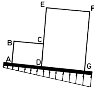
Contraintes inégales imposées au sol et tassements inégaux
