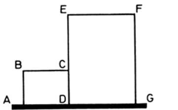
Contraintes inégales imposées au sol et tassements inégaux
