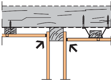
Raccord en angle plafond horizontal ou rampant cf. page 19
