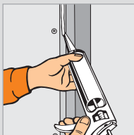
Figure 12 : Etape 2 Appliquer ensuite un cordon de colle FERMACELL sur le chant de la plaque.
