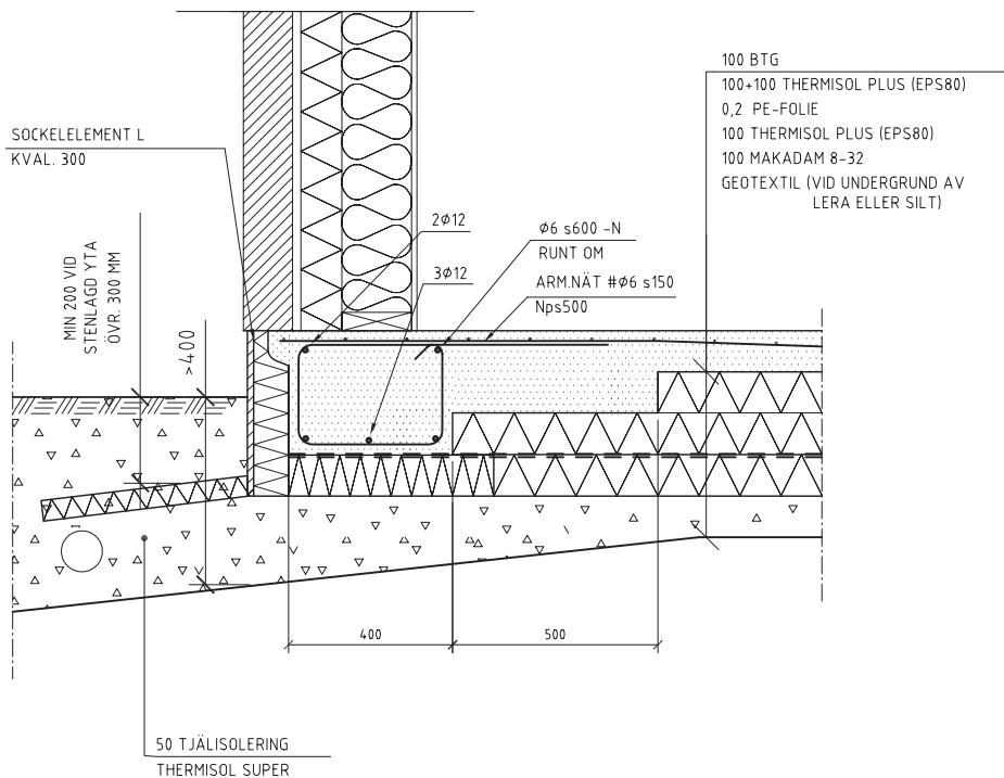
SEKTION A 1:20
