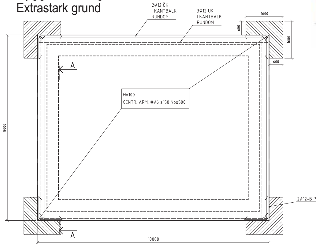
GRUNDPAN 1:100
