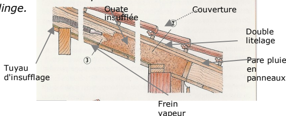
Les schémas sont extraits du merveilleux livre de JP Oliva "l'isolation écologique, éditions terre vivante"
